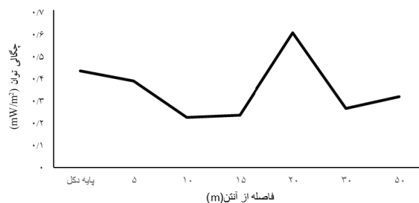
نمودار ۳- مقایسه خطی میانگین چگالی توان امواج همراه اول در زمان‌های آرام و در فواصل مختلف
