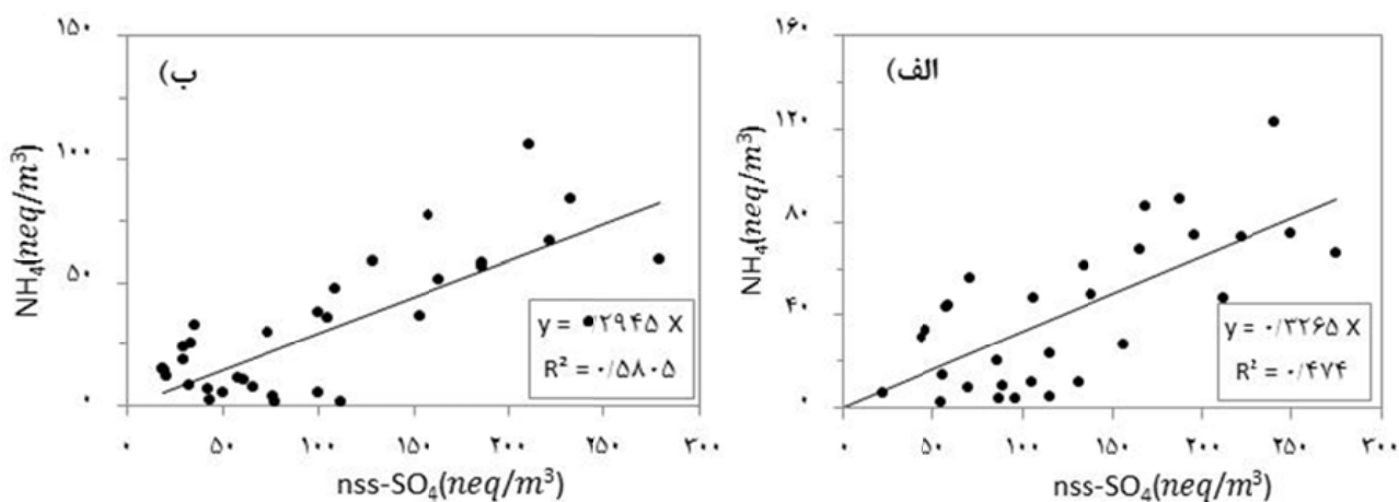
نمودار ۳- ارتباط بین غلظت‌های اکسی‌والانی سولفات ( nss-SO_4 ) و یون آمونیوم در ذرات الف (TSP و ب) PM_{10}
