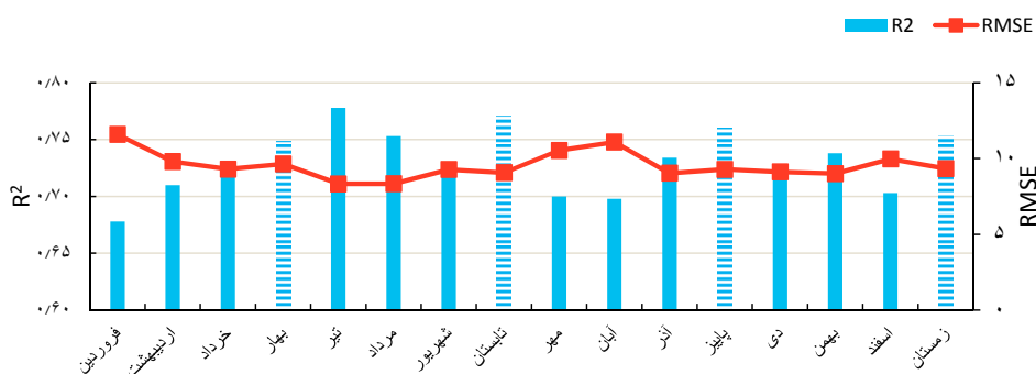
نمودار ۲- نتایج مدلسازی غلظت ازن برحسب ppb
