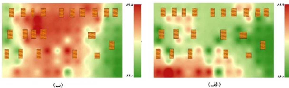
شکل ۷- (الف) تراز فشار صوت اولیه، (ب) تراز فشار صوت بعد از جابه‌جایی دستگاهها
