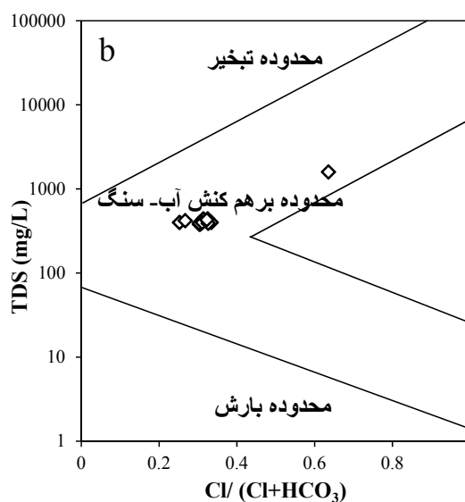
نمودار ۲- نمودارهای گیس آب چاه نیمه‌ها الف) شهریور ۹۶ ب) فروردین ۹۷
