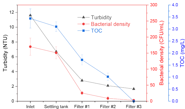
نمودار ۴- میانگین حذف TOC و عوامل میکروبی در واحد فیلتر اسفنجی بافل دار (در کدورت ۱۰ NTU و بار سطحی ۱۰ m/h)
