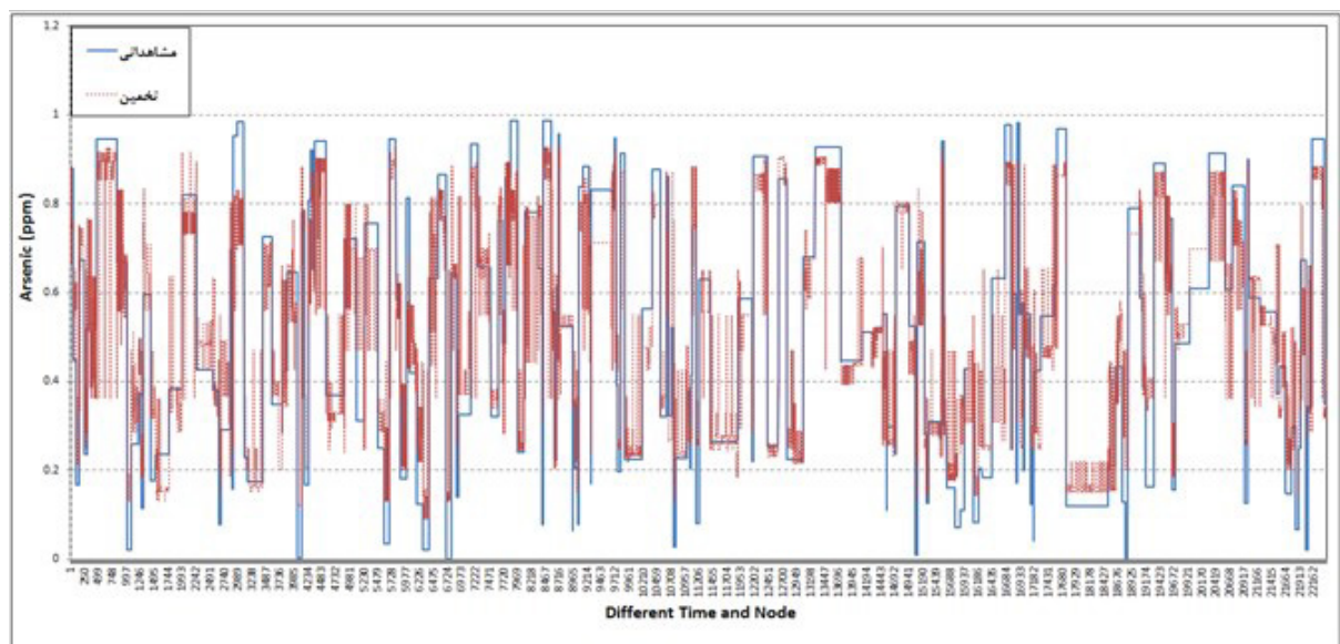
شکل ۶- مقایسه مقادیر آلودگی پیش‌بینی شده و مشاهداتی در ۲۲۳۹۸ نقطه شبکه توزیع آب تحت پوشش مخزن ۴
