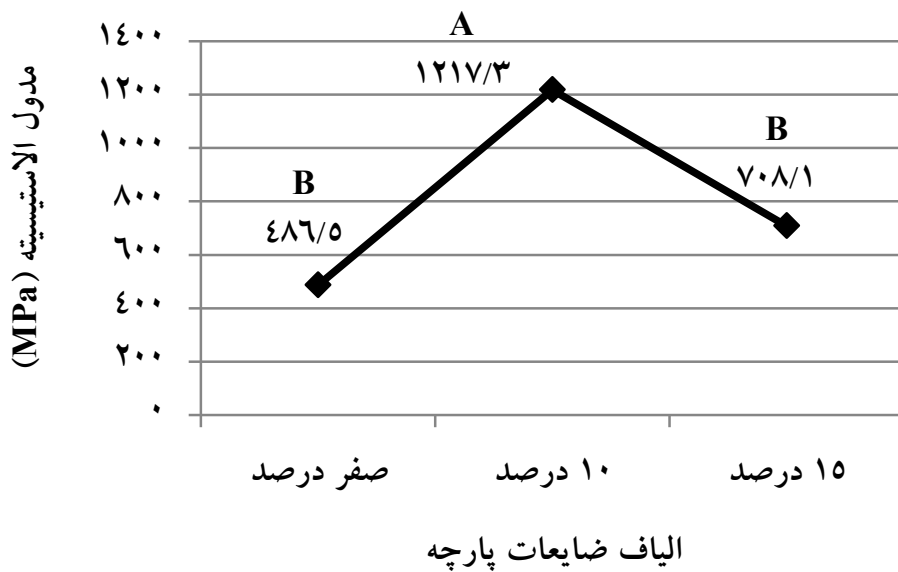
نمودار ۲- اثر استفاده از الیاف ضایعات پارچه بر مدول الاستیسیته تخته فیبرهای ساخته شده
