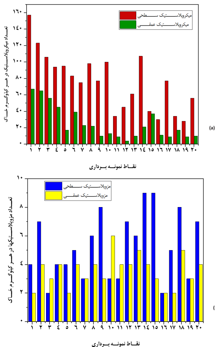
نمودار ۱- مقایسه فراوانی میکرو و مزوپلاستیک در خاک سطحی و عمقی منطقه مسکونی
