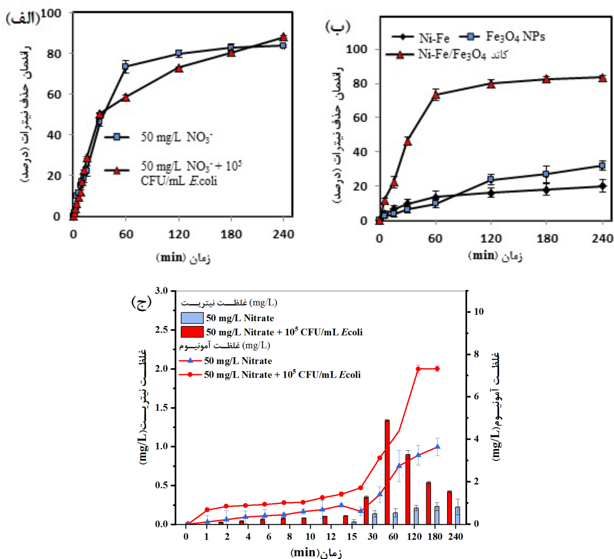
نمودار 2- (الف) اثر حضور باكتري اشرشياكلى بر راندمان حذف نيترات، (ب) سهم اجزای الكترود بر راندمان حذف نيترات و (ج) غلظت نيتريت و آمونيووم توليدى در فرايند احياى نيترات
