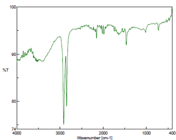
شکل ۳- طیف FTIR شناسایی شده پلی پروپیلن دستگاہ گوارش میگوی وانامی
