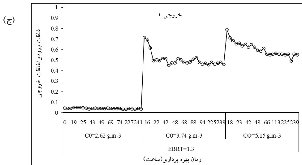
ادامه نمودار ۱- نسبت C/C_0 در EBRTs و غلظت‌های مختلف در خروجی ۱
