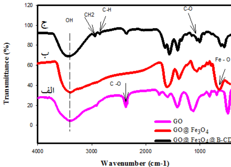
شکل ۳- طیف FT-IR از گرافن اکساید (الف)، گرافن اکساید مغناطیسی (ب) و گرافن اکساید مغناطیسی عامل‌دار شده با \beta سیکلودکسترن (ج)
