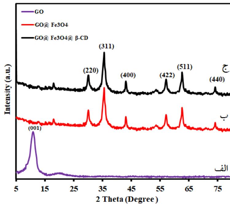
شکل ۲- طیف XRD از گرافن اکساید (الف)، گرافن اکساید مغناطیسی (ب) و گرافن اکساید مغناطیسی عامل‌دار شده با \beta سیکلودکسترن (ج)
