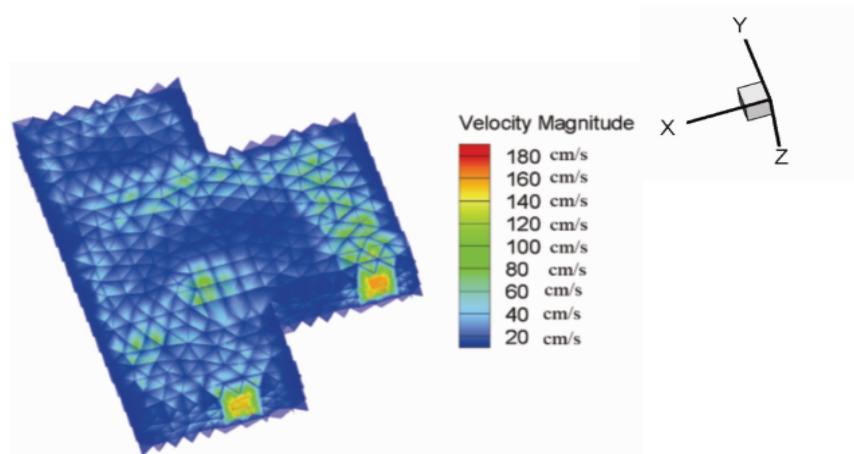
شکل ۷: هم مقدارهای سرعت در محیط بسته بر حسب سانتی متر بر ثانیه
