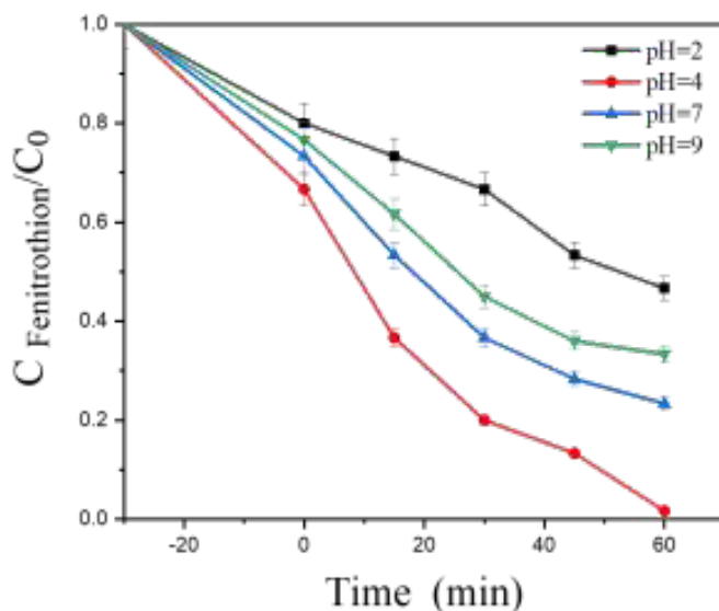
شکل ۵- تاثیر pH اولیه محلول (الف)، غلظت فوتوکاتالیست (ب) و زمان تماس (ج) بر نرخ حذف فنیتروتیون توسط GO@Fe_3O_4 ، GO@Fe_3O_4/CeO_2 (غلظت اولیه فنیتروتیون = 30 \text{ mg/L} ، غلظت فوتوکاتالیست = 20 \text{ mg/L} و \text{pH} = 7 )
