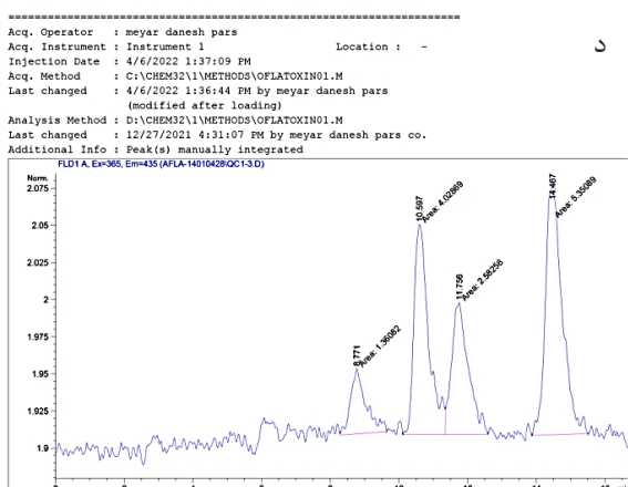
شکل ۱- کروماتوگرام های استاندارد الف) داکسی نیوالول با غلظت ۱۰۰۰ µg/L (ب) زیرالنون با غلظت ۱۰۰ µg/L (ج) اکراتوکسین با غلظت ۵ µg/L (د) استاندارد آفلاتوکسین ها با غلظت ۱ µg/L
