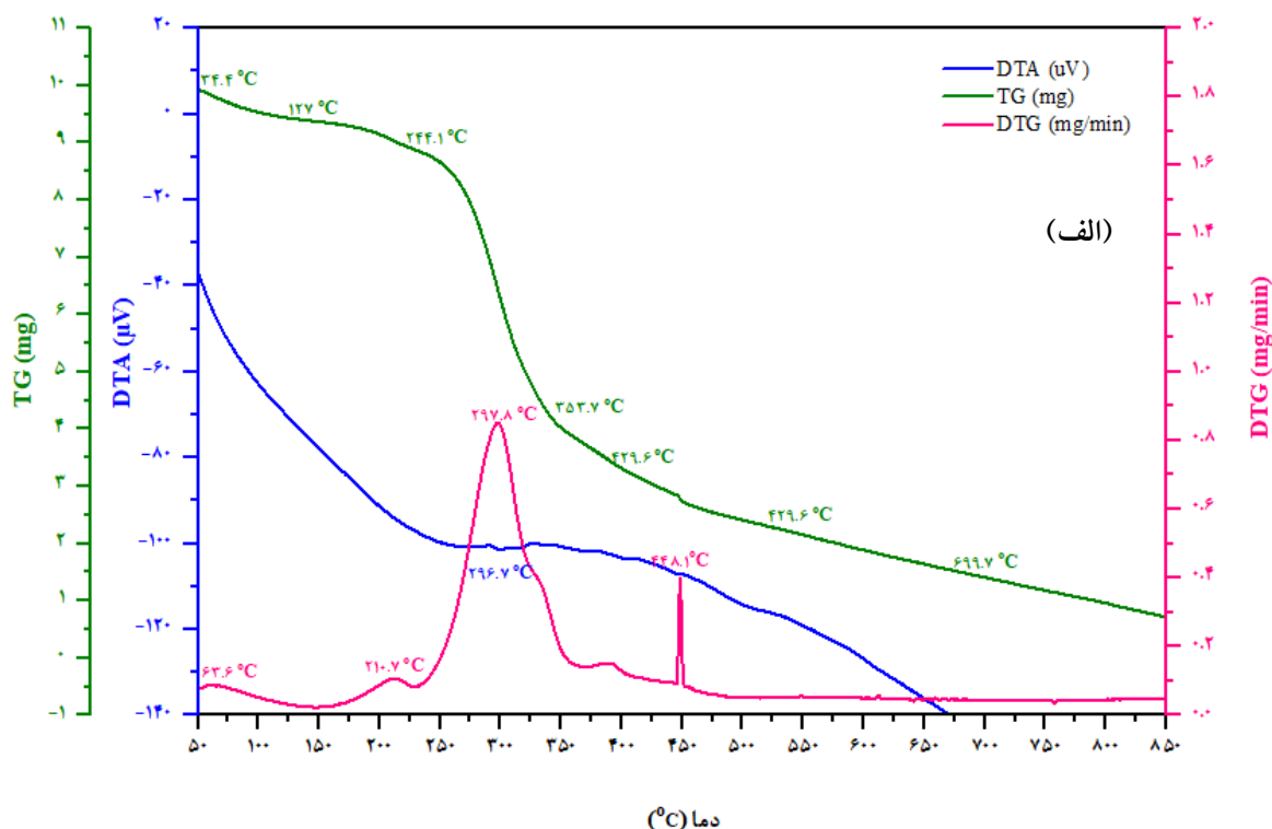
نمودار ۳- منحنی آنالیز توزین حرارتی الف) SCG و ب) هیدروچار حاصله در شرایط بهینه ( 235^\circ\text{C} ، 180 \text{ min} و نسبت (۸:۱) L:S
