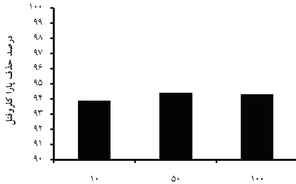
شکل ۴: مقایسه راندمان حذف در غلظت های ۱۰، ۵۰ و ۱۰۰ میلی گرم بر لیتر توسط فرایند شبه فنتون ( H_2O_2 /para-cp=18/8 H_2O_2 /Fe 0 =0/4)
