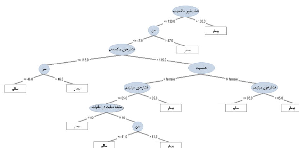
شکل شماره ۲- درخت تصمیم با رویکرد هزینه‌محور بر روی مجموعه داده بدون در نظر گرفتن مشخصه‌های هزینه‌ها
