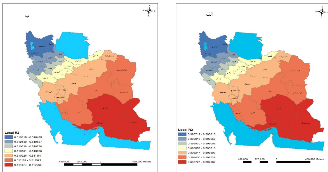
شکل شماره 2- مقادیرهای محلی در (الف) زنان (ب) مردان در ایران، سال 1388
