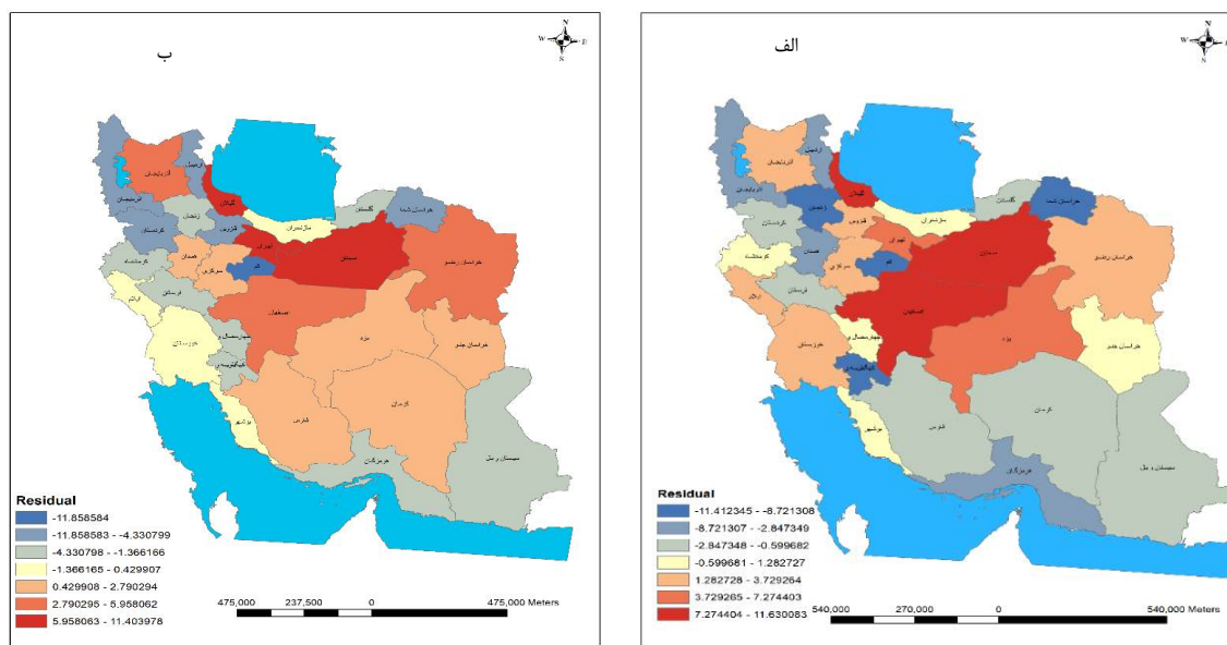
شکل شماره 1- مقادیرهای باقی مانده تفاضل بین مقادیرهای مشاهده شده و مقادیرهای برآورده شده در (الف) زنان (ب) مردان در ایران، سال 1388
