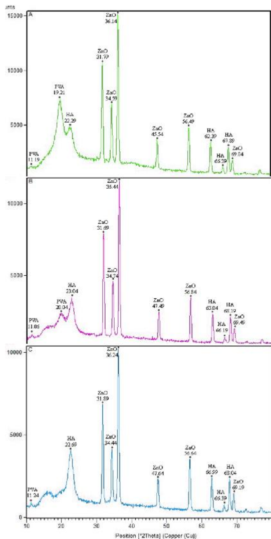
شکل ۴: آنالیز پراش تفرقی اشعه ی ایکس (XRD) فیلم های: A) 85%PVA-10%HA-5%ZnO (B) 70%PVA-20%HA-10%ZnO (C) و 55%PVA-30%HA-15%ZnO
