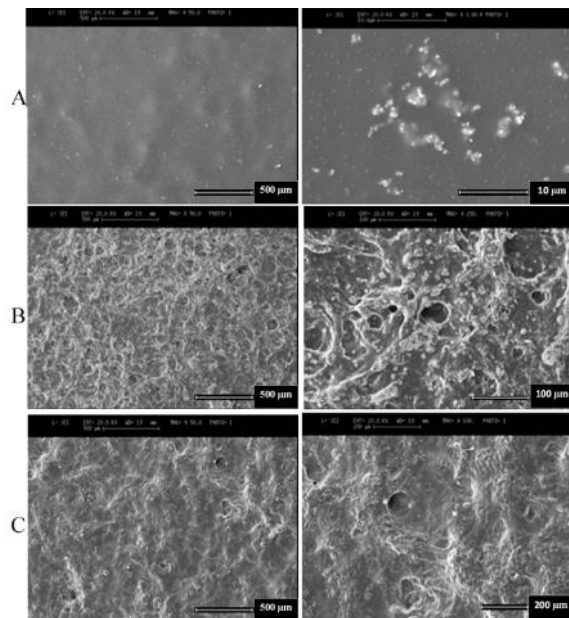
شکل ۳: تصویر میکروسکوپ SEM از فیلم های: A) 85%PVA-10%HA-5%ZnO (B) 70%PVA-20%HA-10%ZnO (C) و 55%PVA-30%HA-15%ZnO
