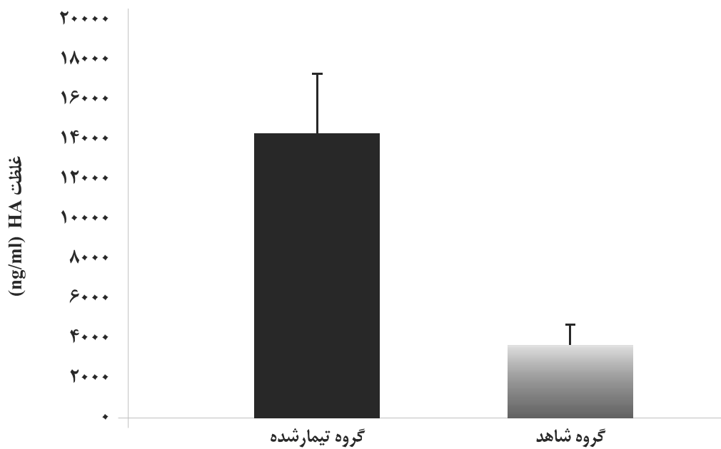
شکل ۸: نمودار میزان ترشح HA. میانگین ترشح HA در گروه تیمار شده، 3/96 \pm 0/39 برابر گروه شاهد است با دارا بودن P=0/0001
