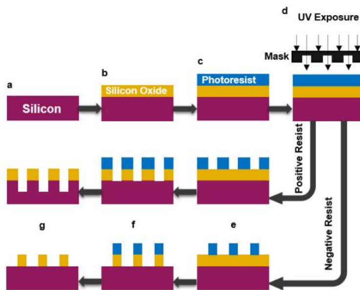
شکل ۵: فرآیند لیتوگرافی ۲۵ .
