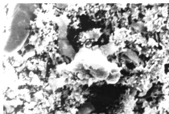
شکل ۱۲- نمای SEM گروه MTA سفید روز هفتم بزرگنمایی \times 1000 اتصال سلولی قابل مشاهده است.
