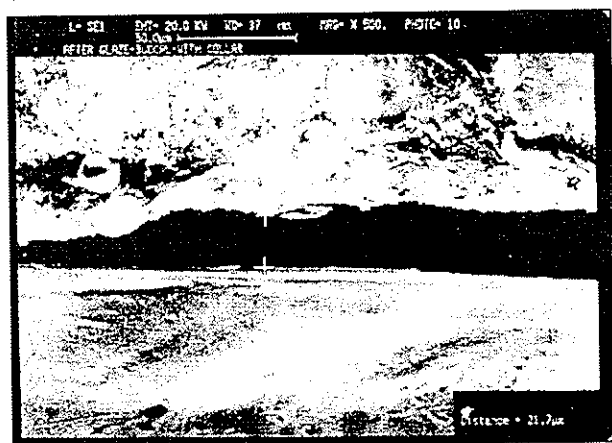
تصویر شماره ۳- سطح باکال در نمونه با کلار با بزرگنمایی ۵۰۰ برابر در مرحله بعد از گلایز
