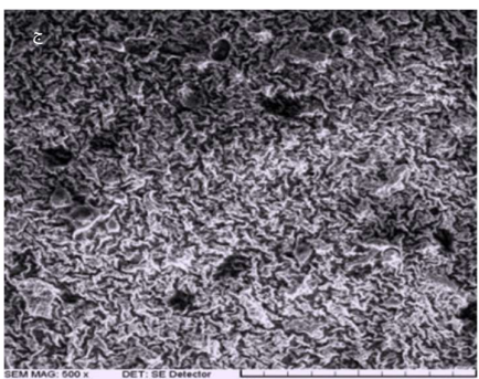
شکل ۳- مورفولوژی اکسیدهای سطحی بعد از گاز زدایی در آلیاژهای Verabond (الف)، Damcast (ب) و Noritake (ج)
