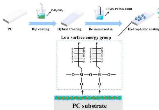
شکل ۲- شماتیک پوشش سل‌ژل هیبریدی زیرکونیا/سیلیکا همراه با لایه نهایی با انرژی سطحی پایین (۱۱)
