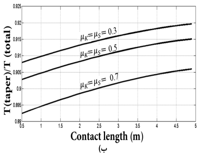
شکل ۹- نسبت گشتاور مخروط به گشتاور کل برحسب ضریب اصطکاک استاتیکی، ب) سطح تماس مخروط
