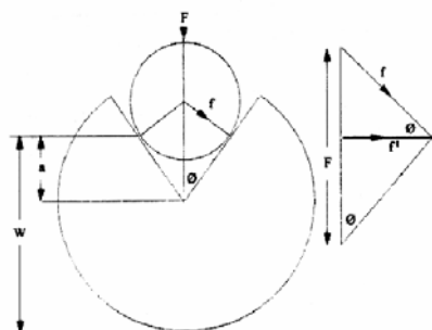
شکل ۳- نمایشی از نحوه اعمال نیرو برای محاسبه K_{IC}
