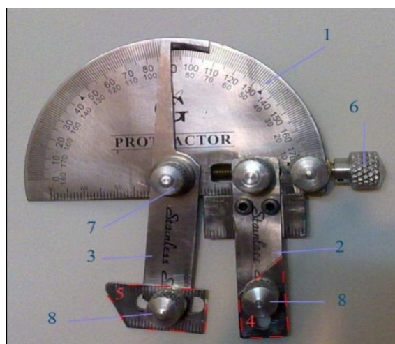
شکل 1- اجزای تشکیل دهنده وسیله: 1- صفحه مدرج 2- بازوی با محور ثابت 3- بازوی با محور متحرک 4- زاویه تنظیم طول بازوی با محور ثابت 5- زاویه تنظیم فاصله بین دو بازو در صورت لزوم 6- پیچ تنظیم کننده فاصله بین دو بازو 7- پیچ تنظیم کننده بازوی با محور متحرک 8- پیچ های تنظیم کننده زاویه ها
