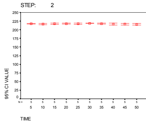
نمودار ۱- اطمینان ۹۵٪ در پله دوم با تغییر زمان تابش الف- نمودار رابطه میزان Pixel value را با افزایش زمان تابش در پله دوم نشان می‌دهد.
