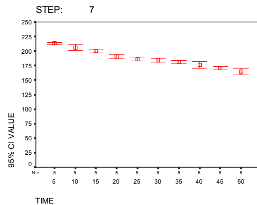
ب- نمودار رابطه میزان Pixel value را با افزایش زمان تابش در پله هفتم نشان می‌دهد.
