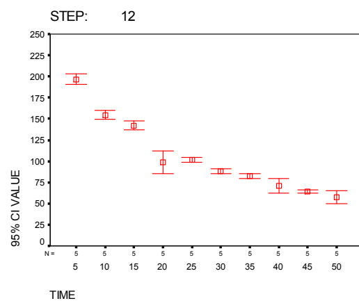
ج- نمودار رابطه میزان Pixel value را با افزایش زمان تابش در پله دوازدهم نشان می‌دهد.
