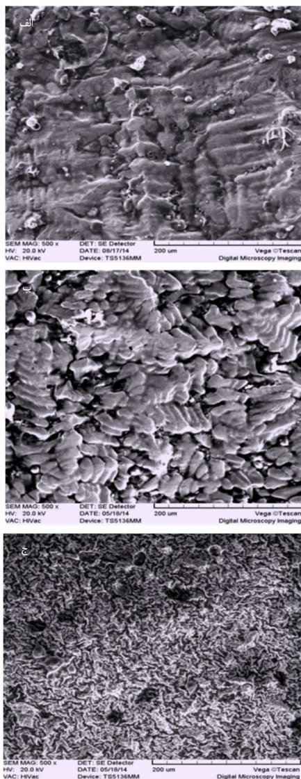
شکل ۳- مورفولوژی اکسیدهای سطحی بعد از گاز زدایی در آلیاژهای Verabond (الف)، Damcast (ب) و Noritake (ج)
