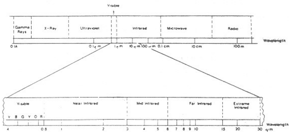
شکل ۴ - طیف الکترومغناطیس
