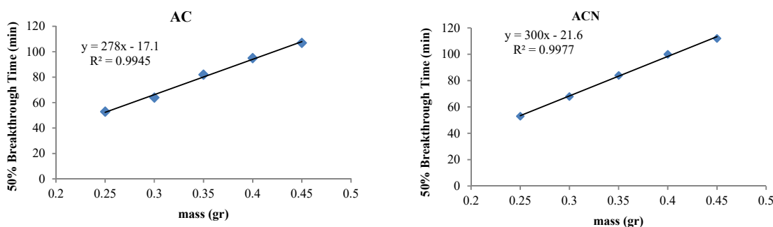
شکل (7) - نمودار زمان نقطه شکست 50 درصد سووفلوران روی جاذب های AC و ACN در مقابل جرم
