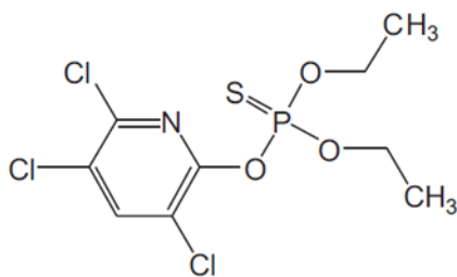
شکل ۱: ساختار کلرپیریفوس
