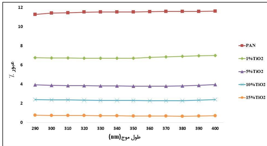
شکل ۳. درصد عبور تابش فرابنفش از نمونه های مختلف نانوالیاف الکتروسی شده
