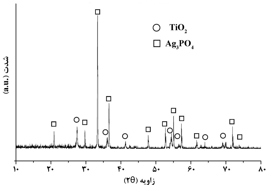
شکل ۲. الگوی پراش اشعه ایکس نمونه \text{Ag}_3\text{PO}_4/\text{TiO}_2
