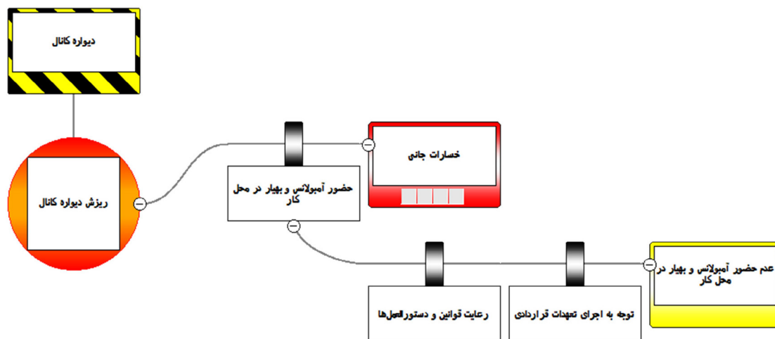
شکل ۱۶: نمودار Bowtie برای فاکتور تشدید کننده حضور آمبولانس و بهیبار در محل کار در حوادث ریش دیواره کانال در عملیات گودبرداری و لوله‌گذاری خطوط لوله گاز
