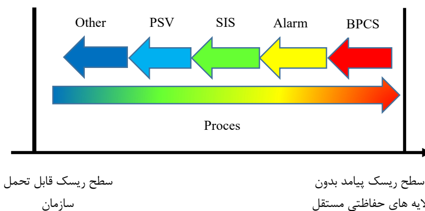
شکل ۲: لایه های حفاظتی مستقل در واحد های صنعتی (۴، ۲).
