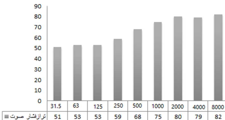
شکل ۲: میانگین تراز فشار صوت ۸۵ دسی بل در فرکانس های مرکزی یک اکتاوباند در ۲۱ روز مواجهه با صدا ( مدت زمان آزمایش: ۳۰ روز)
