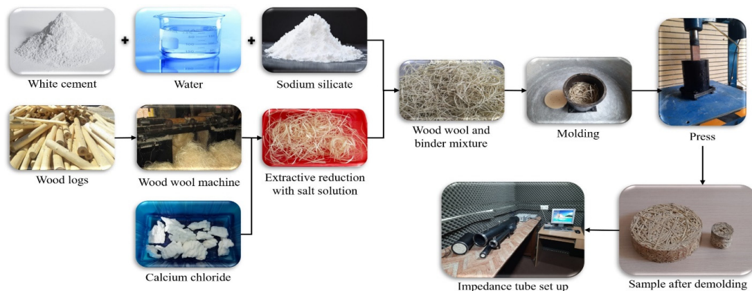
شکل ۱: فلوچارت ساخت نمونه‌ها و اندازه‌گیری ضریب جذب
