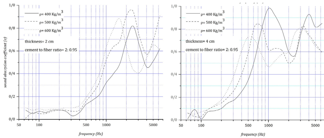
شکل ۳: تاثیر دانسیته الک بر ضریب جذب نمونه‌های WWCP با CFR ۲:۰.۹۵
