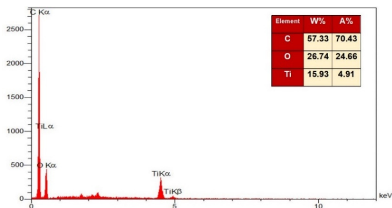
شکل ۶: طیف EDX ابروژل \text{RGO}/\text{CNT}5\%/\text{TiO}_2
