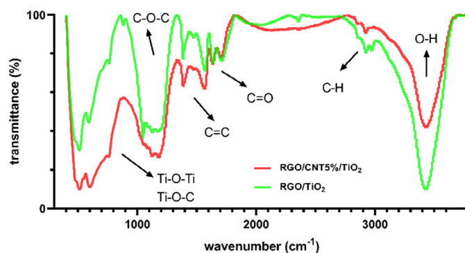
شکل ۵: طیف FT-IR ابروژل \text{RGO}/\text{TiO}_2 و \text{RGO}/\text{CNT}5\%/\text{TiO}_2
