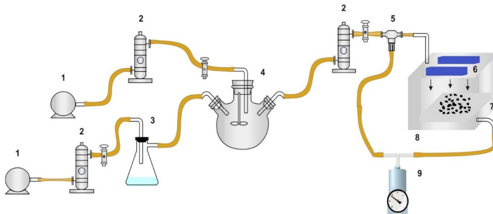
شکل ۲: طرح سیستم فتوکاتالیستی متشکل از: (۱) پمپ هوا، (۲) روماتر، (۳) ظرف حاوی محلول تولوئن، (۴) محفظه اختلاط، (۵) شیشه نمونه‌برداری، (۶) لامپ UV، (۷) ایروژل، (۸) راکتور فتوکاتالیستی، (۹) پورت اندازه‌گیری غلظت تولوئن
