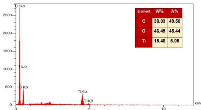
شکل ۷: طیف EDX ابروژل \text{RGO}/\text{TiO}_2
