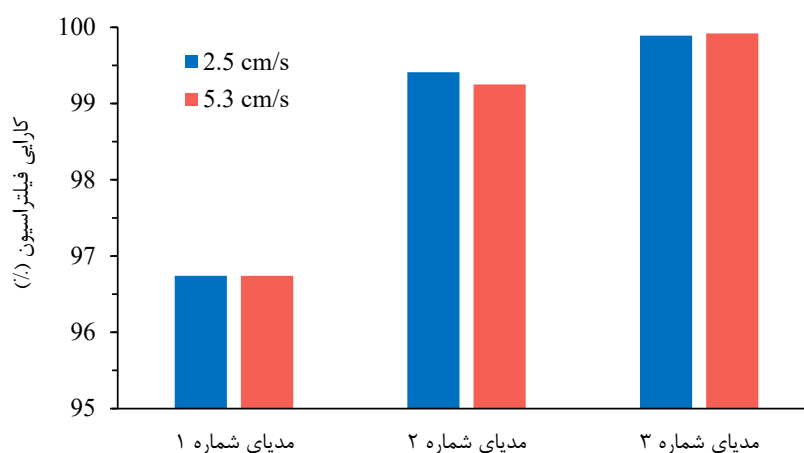
شکل ۳: مقایسه کارایی فیلتراسیون مایه‌های نانولیفی تولید شده با روش الکترورسی محلول در رایش ذرات ۰/۳ میکرون در دو سرعت جریان هوای ۵/۳ و ۲/۵ cm/s
