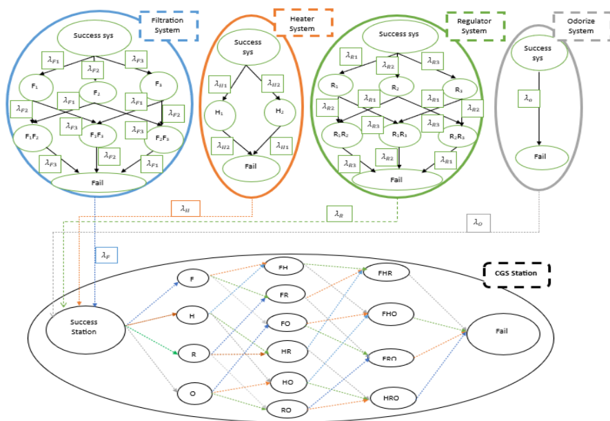
Success Station: موفقیت هر چهار بخش ایستگاه، F: شکست بخش فیلتراسیون، H: شکست بخش گرمکن، R: شکست بخش تقلیل فشار، O: شکست بخش بودار کننده، \lambda_F : نرخ شکست بخش فیلتراسیون، \lambda_H : نرخ شکست سیستم گرمکن، \lambda_R : نرخ شکست بخش تقلیل فشار، \lambda_O : نرخ شکست بخش بودار کننده، Fail: شکست هر چهار بخش ایستگاه
