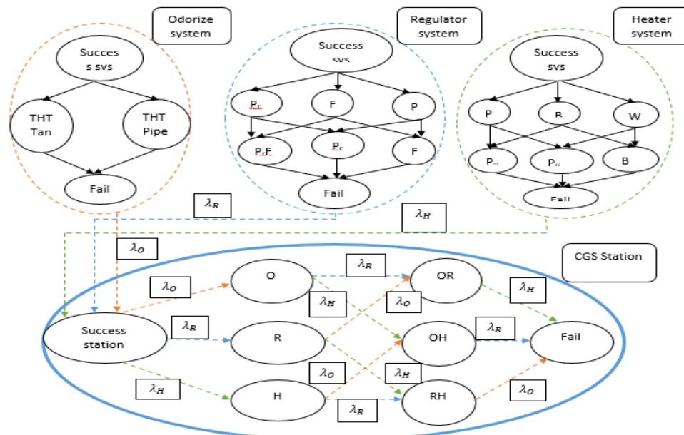
شکل ۱۲: موفقیت هر سه بخش ایستگاه، THT Tank: شکست زیربخش مخزن بودار کننده، THT Pipe: شکست زیربخش خط لوله مخزن بودار کننده، Pr: شکست زیربخش تقلیل فشار، F: شکست زیربخش فیلتراسیون، P: شکست زیربخش پاپلوت، Pu: شکست زیربخش پمپ گرمکن، B: شکست زیربخش بویلر گرمکن، Wp: شکست زیربخش خط لوله آب گرمکن، Fail: شکست هر سه بخش ایستگاه
