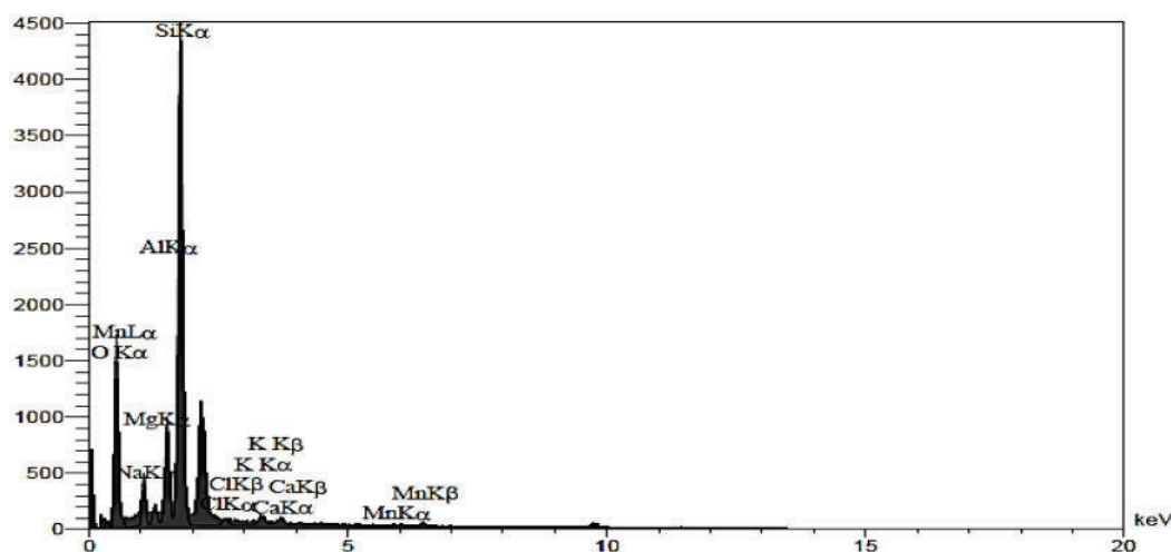
شکل ۳: EDS ژئولیت طبیعی
