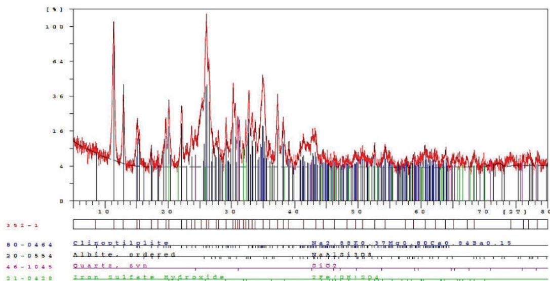
شکل ۴: پراش اشعه ایکس (XRD) ژئولیت طبیعی
