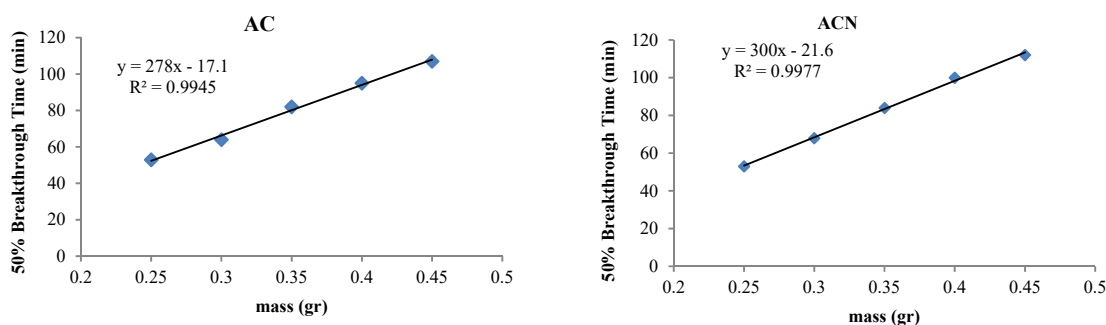
شکل (7) - نمودار زمان نقطه شکست 50 درصد سوئفلوران روی جاذب های AC و ACN در مقابل جرم
