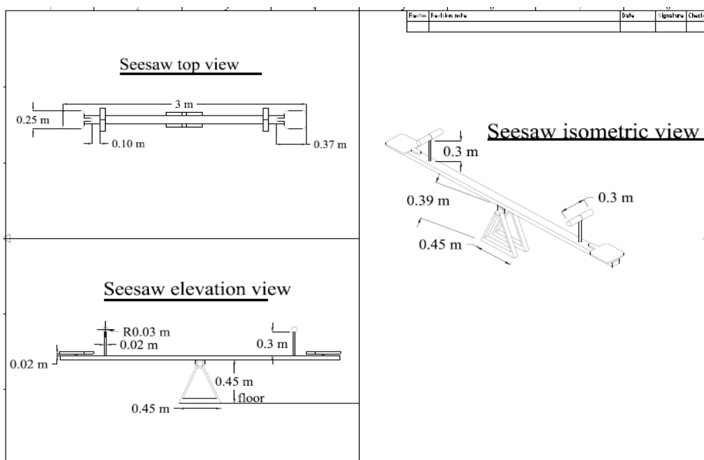
شکل ۳. نقشه طراحی الکلنگ بر اساس داده های آنتروپومتریکی کودکان از نماهای مختلف
