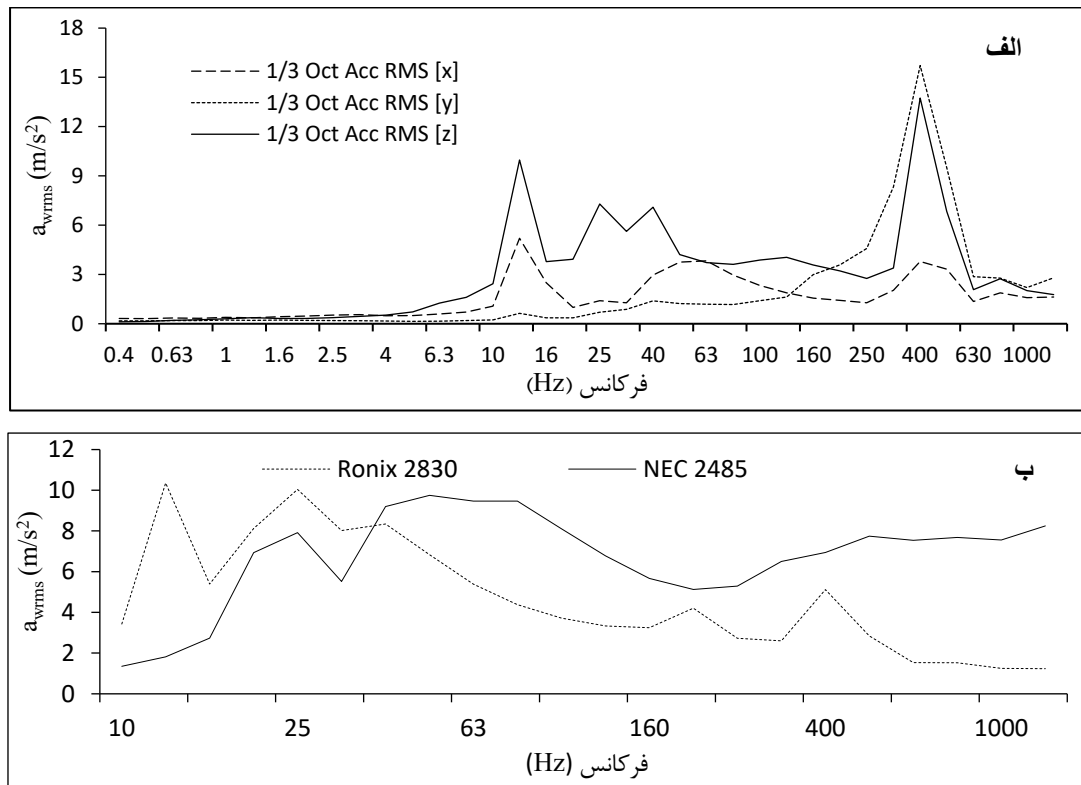
شکل ۷. آنالیز فرکانسی ۱/۳ اکتاو باند به تفکیک محورهای ارتعاشی حین تخریب یک قطعه بتنی با ضخامت ۱۵ cm در دسته راست چکش رونیکس با قلم تخت و طول ۶۰ cm (الف) و میانگین مقادیر ۱/۳ اکتاوباند در طیف فرکانسی w_h هر چکش (ب)
