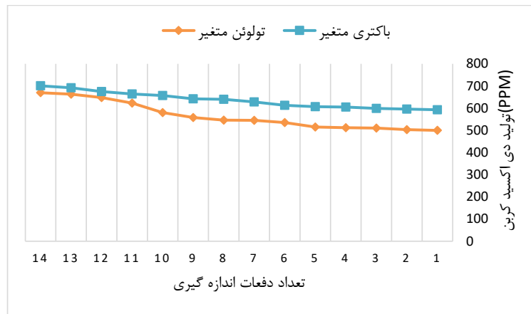
شکل ۴: تولید دی اکسید کربن در شیبه اول (زیست توده متغیر) و شیبه دوم (تولوئن متغیر)
