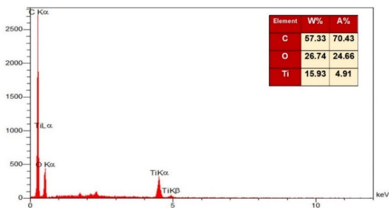
شکل ۶: طیف EDX ایروزل RGO/CNT 5 %/TiO 2
