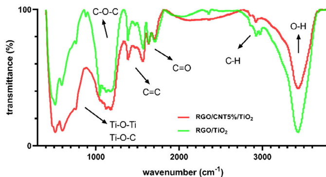
شکل ۵: طیف FT-IR ایروزل RGO/CNT 5 %/TiO 2 و RGO/TiO 2
