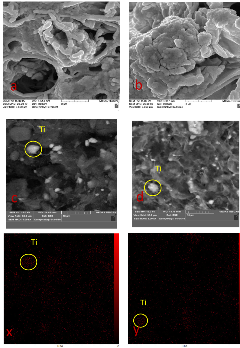
شکل ۳: a و c و x تصویر SEM و EDS-mapping ایروژل \text{RGO/CNT}/5/\text{TiO}_2 و b و d و y تصویر SEM و EDS-mapping ایروژل \text{RGO/TiO}_2
