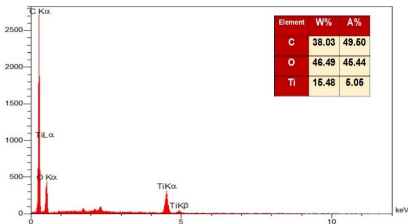
شکل ۷: طیف EDX ایروزل RGO/TiO 2
